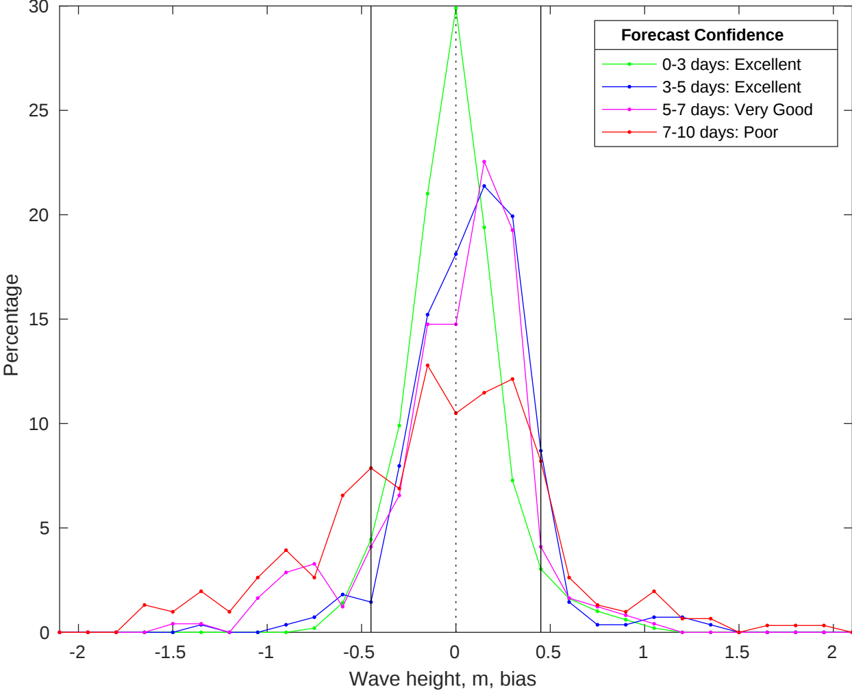
NDBC 46028 vs CMEMS Waves Bias Histogram: 02-Jan-2026
