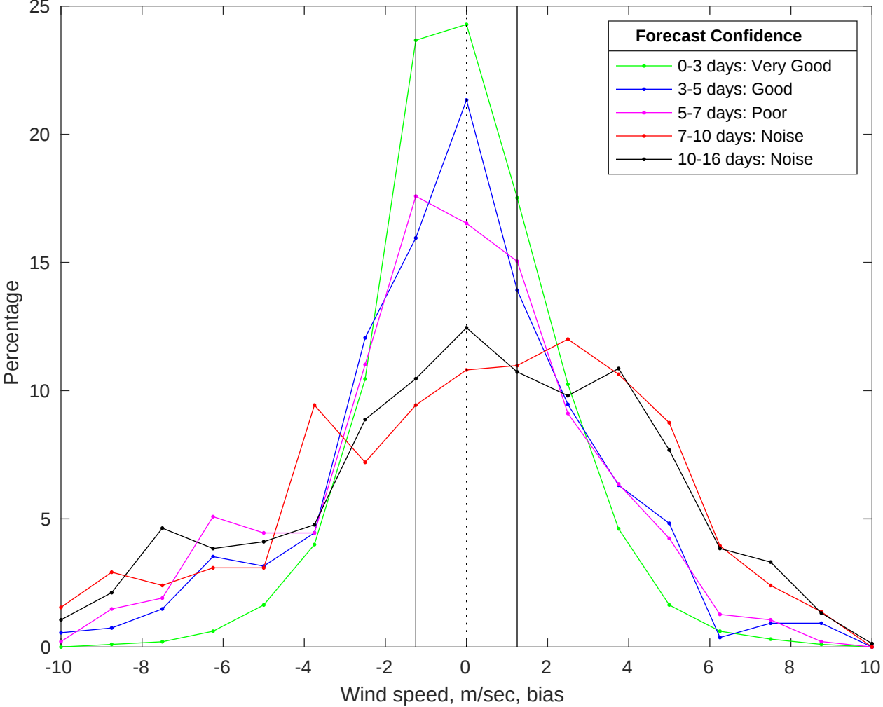
NDBC 46054 vs GFS Winds Bias Histogram: 02-Jan-2026
