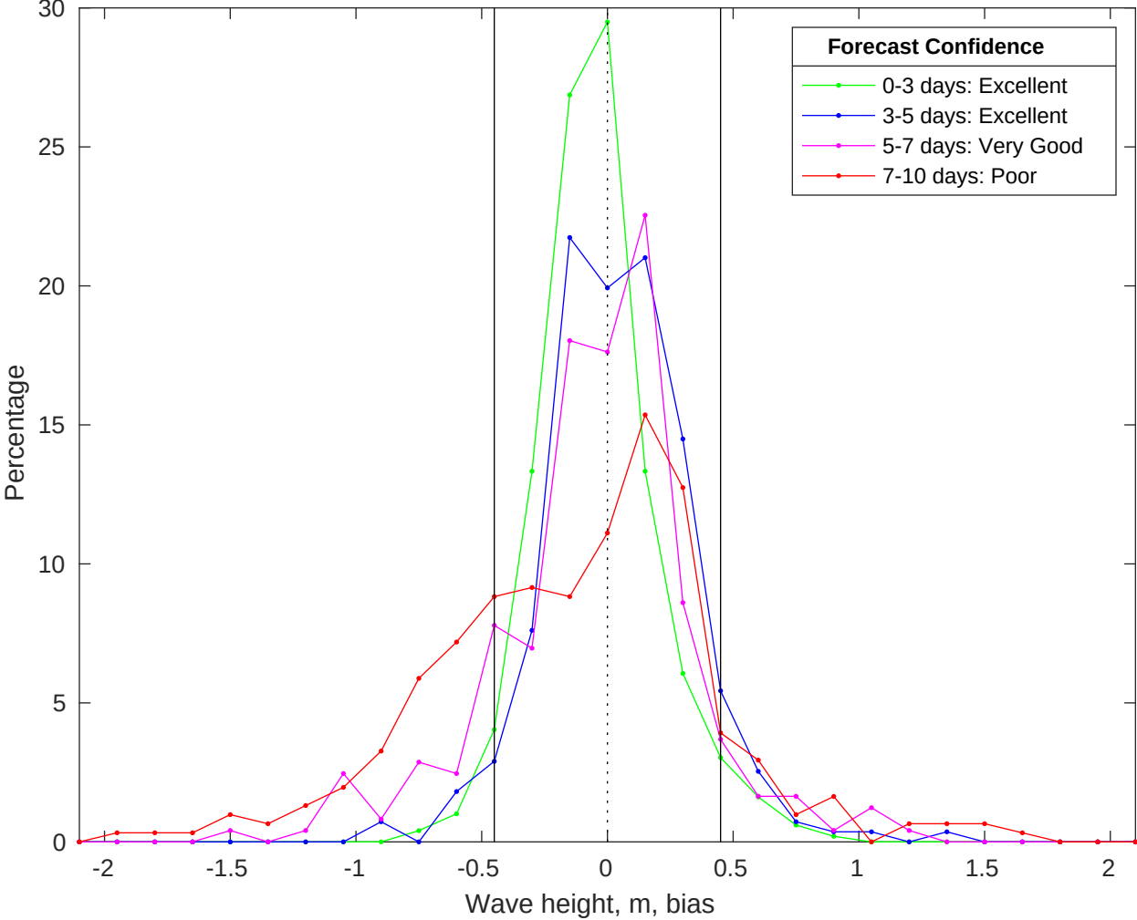
NDBC 46259 vs CMEMS Waves Bias Histogram: 02-Jan-2026
