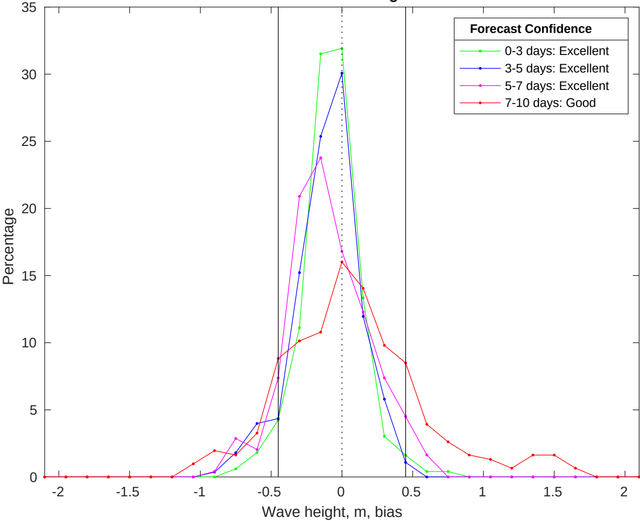
NDBC 51000 vs CMEMS Waves Bias Histogram: 02-Jan-2026
