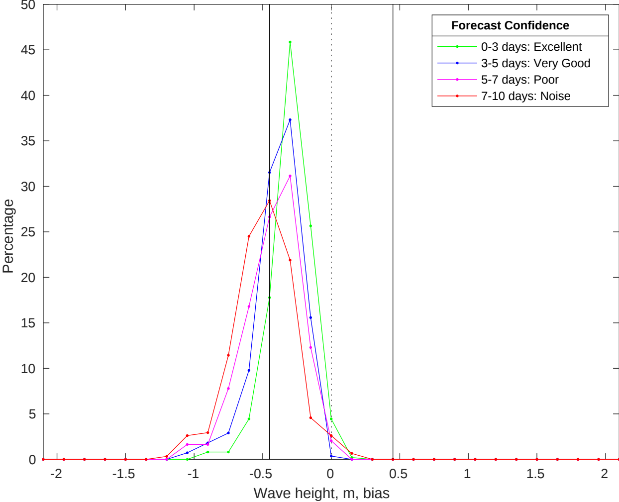
NDBC 51209 vs CMEMS Waves Bias Histogram: 02-Jan-2026
