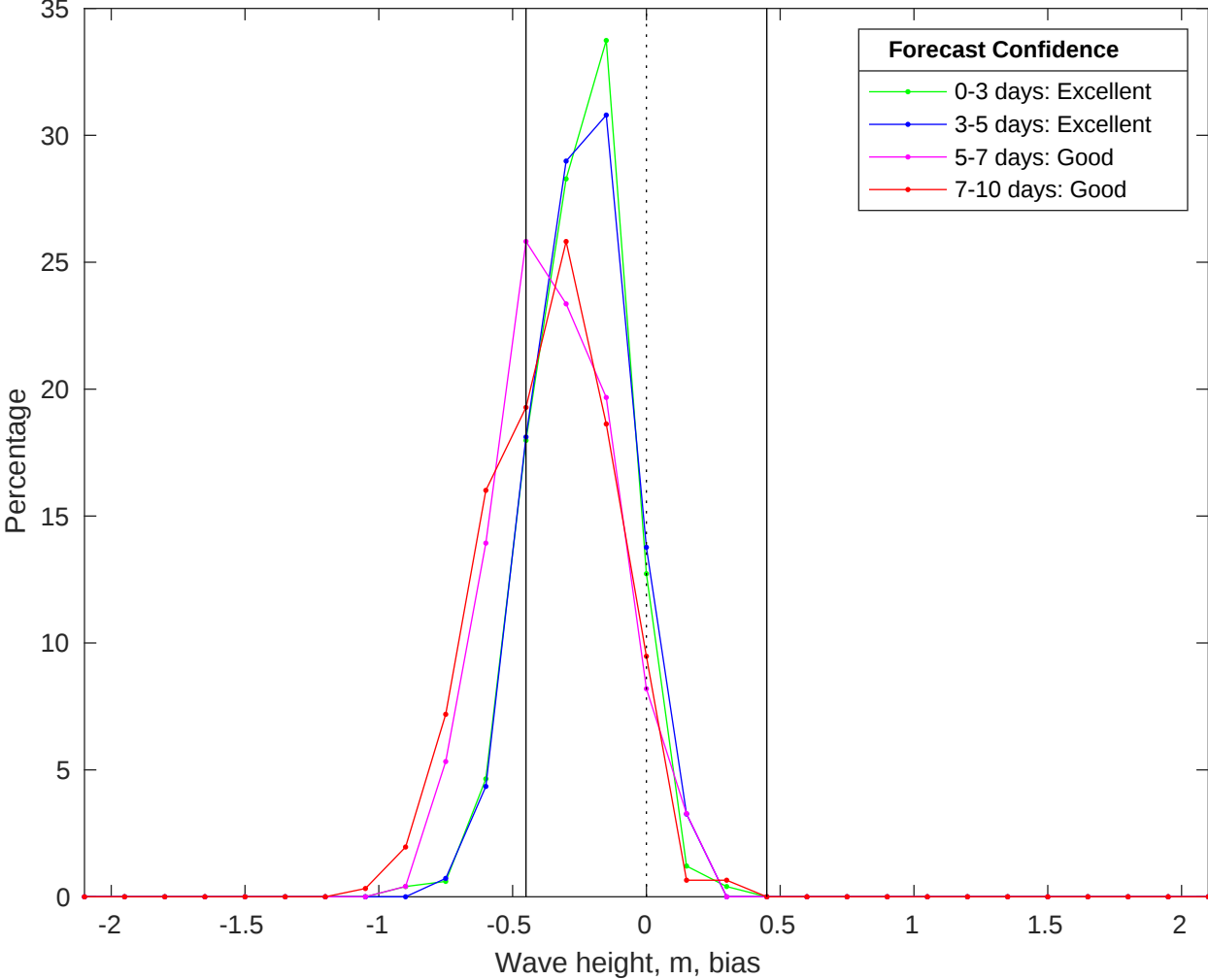
NDBC 52213 vs CMEMS Waves Bias Histogram: 02-Jan-2026
