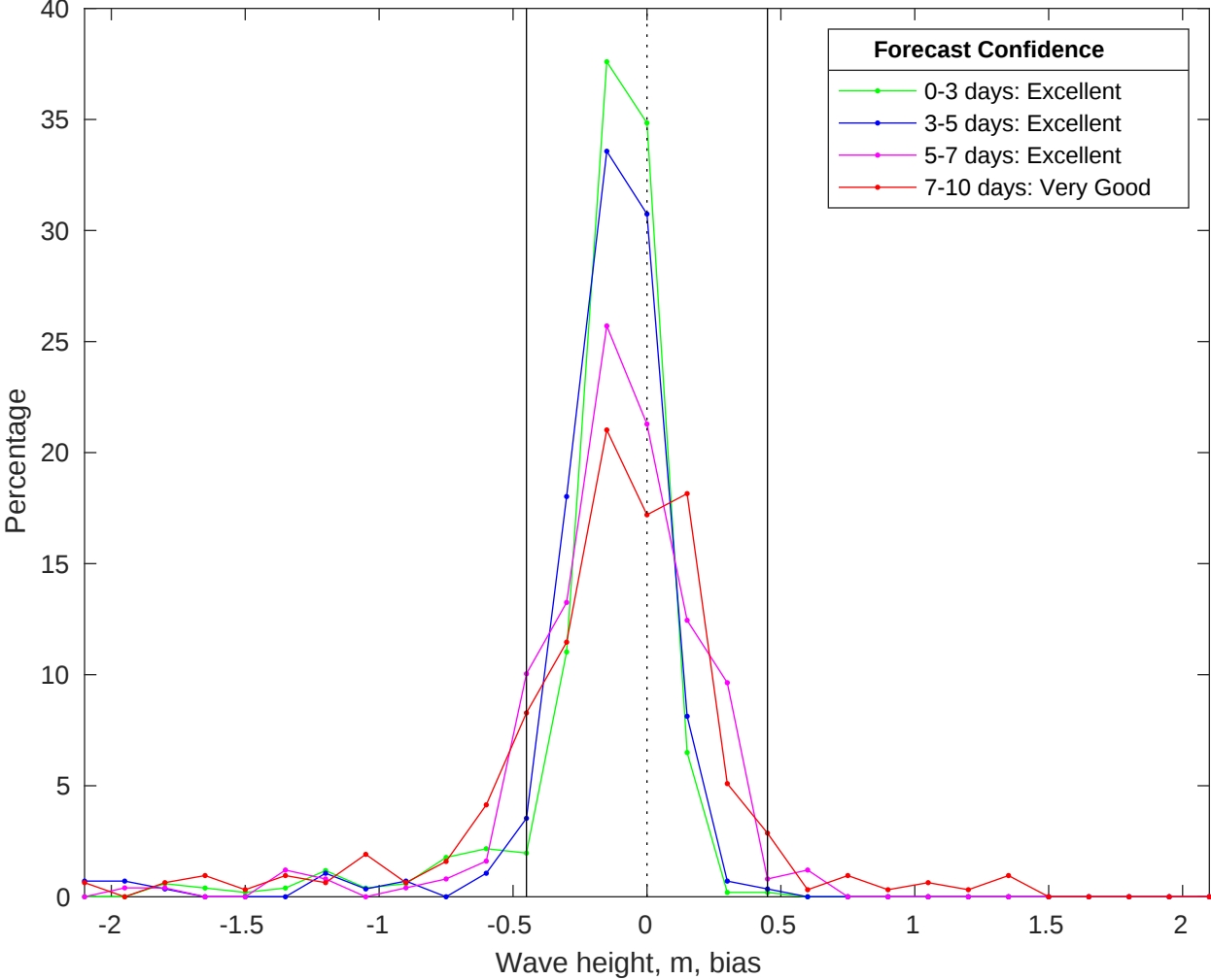
NDBC 42019 vs CMEMS Waves Bias Histogram: 03-Jan-2026
