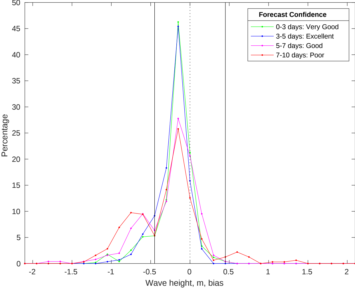
NDBC 42036 vs CMEMS Waves Bias Histogram: 03-Jan-2026
