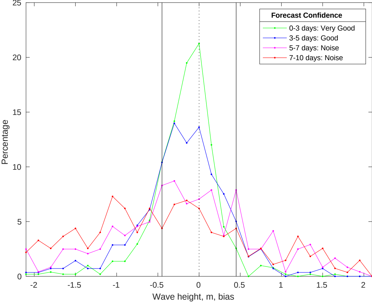
NDBC 44008 vs CMEMS Waves Bias Histogram: 03-Jan-2026
