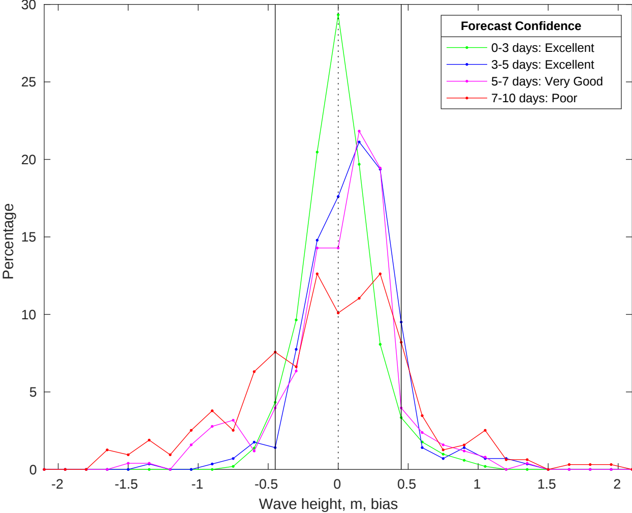
NDBC 46028 vs CMEMS Waves Bias Histogram: 03-Jan-2026
