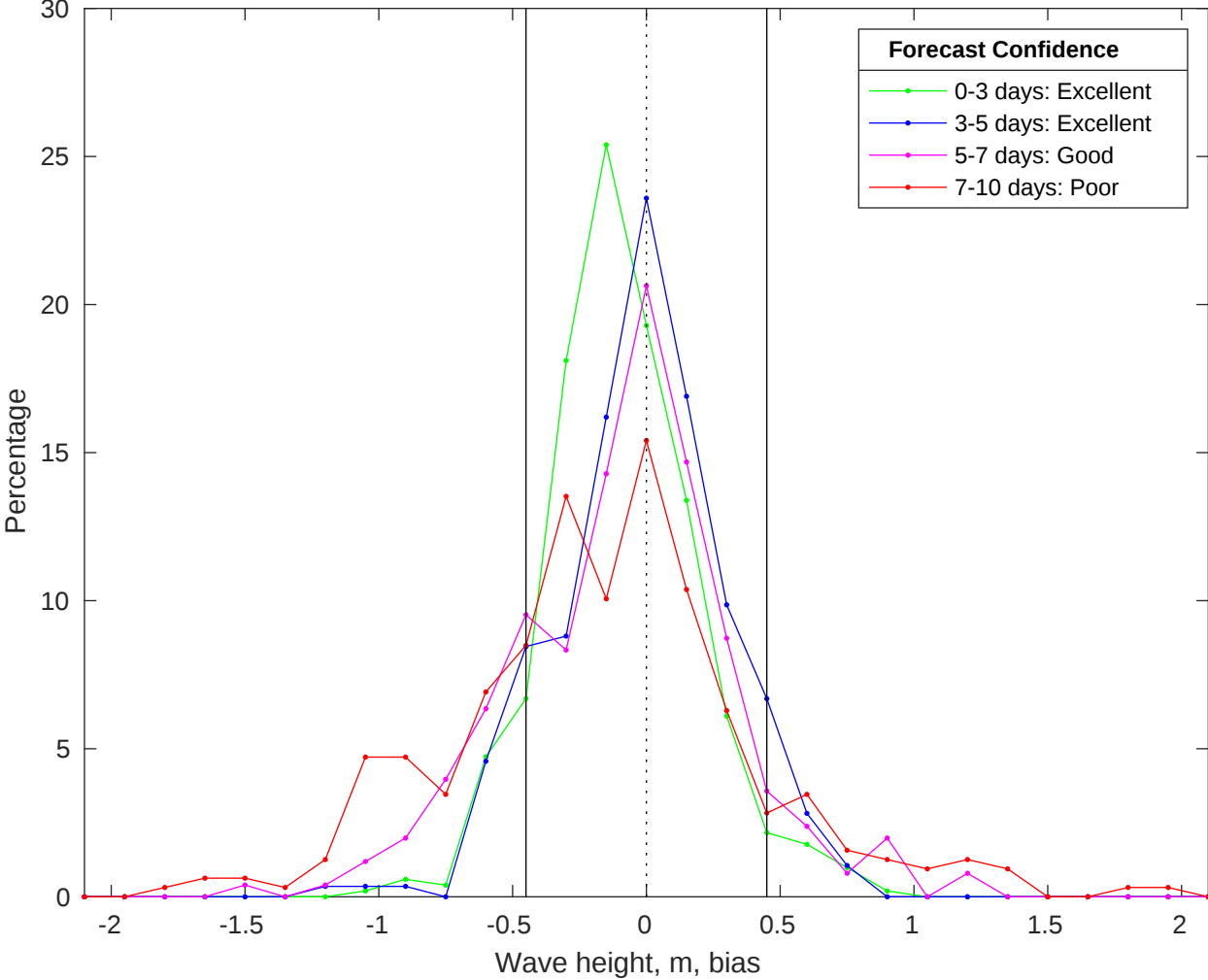
NDBC 46054 vs CMEMS Waves Bias Histogram: 03-Jan-2026
