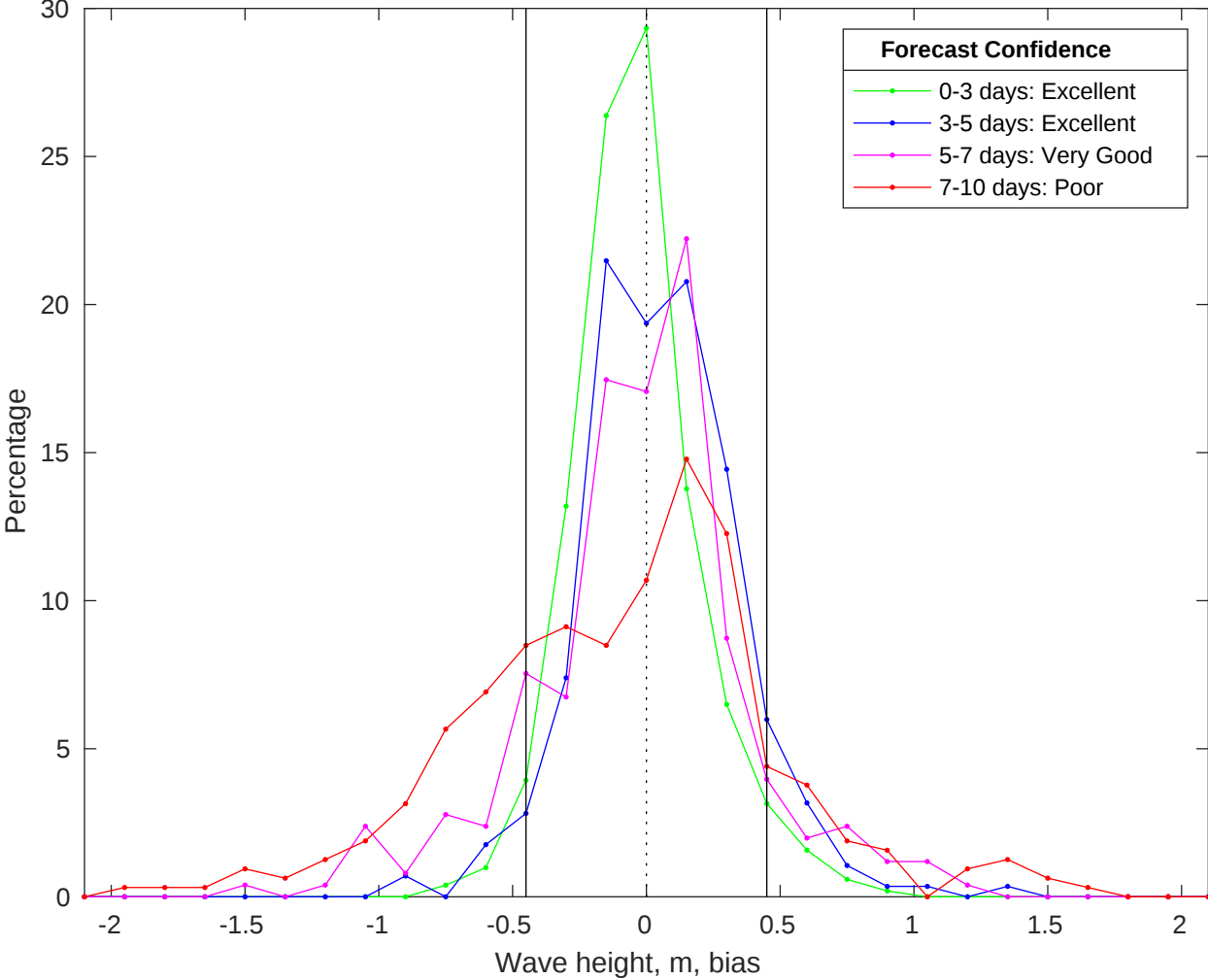
NDBC 46259 vs CMEMS Waves Bias Histogram: 03-Jan-2026
