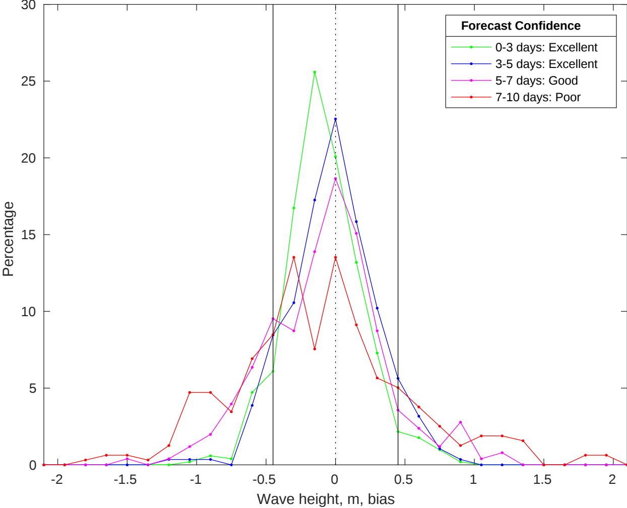
NDBC 46054 vs CMEMS Waves Bias Histogram: 04-Jan-2026
