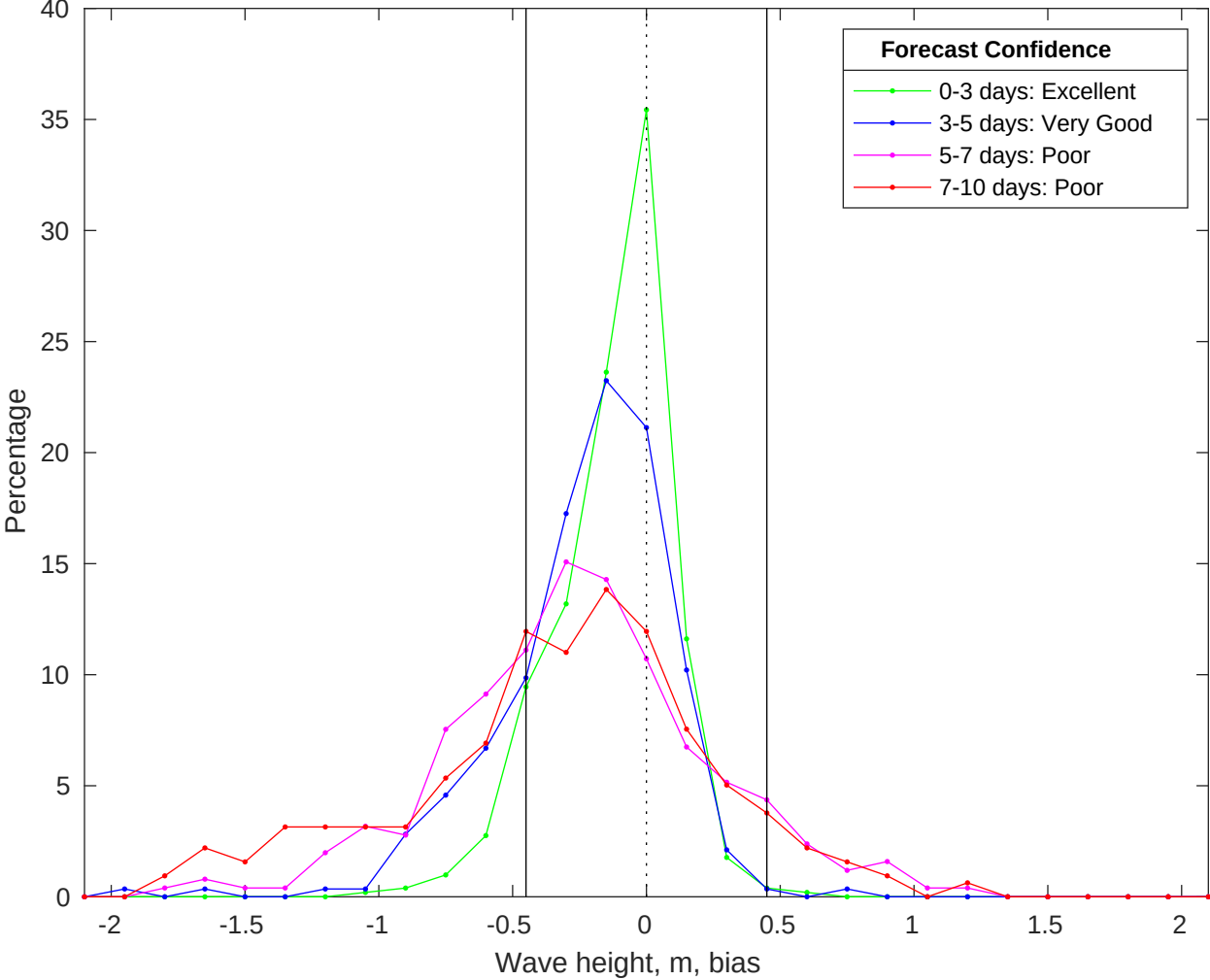
NDBC 41013 vs CMEMS Waves Bias Histogram: 05-Jan-2026
