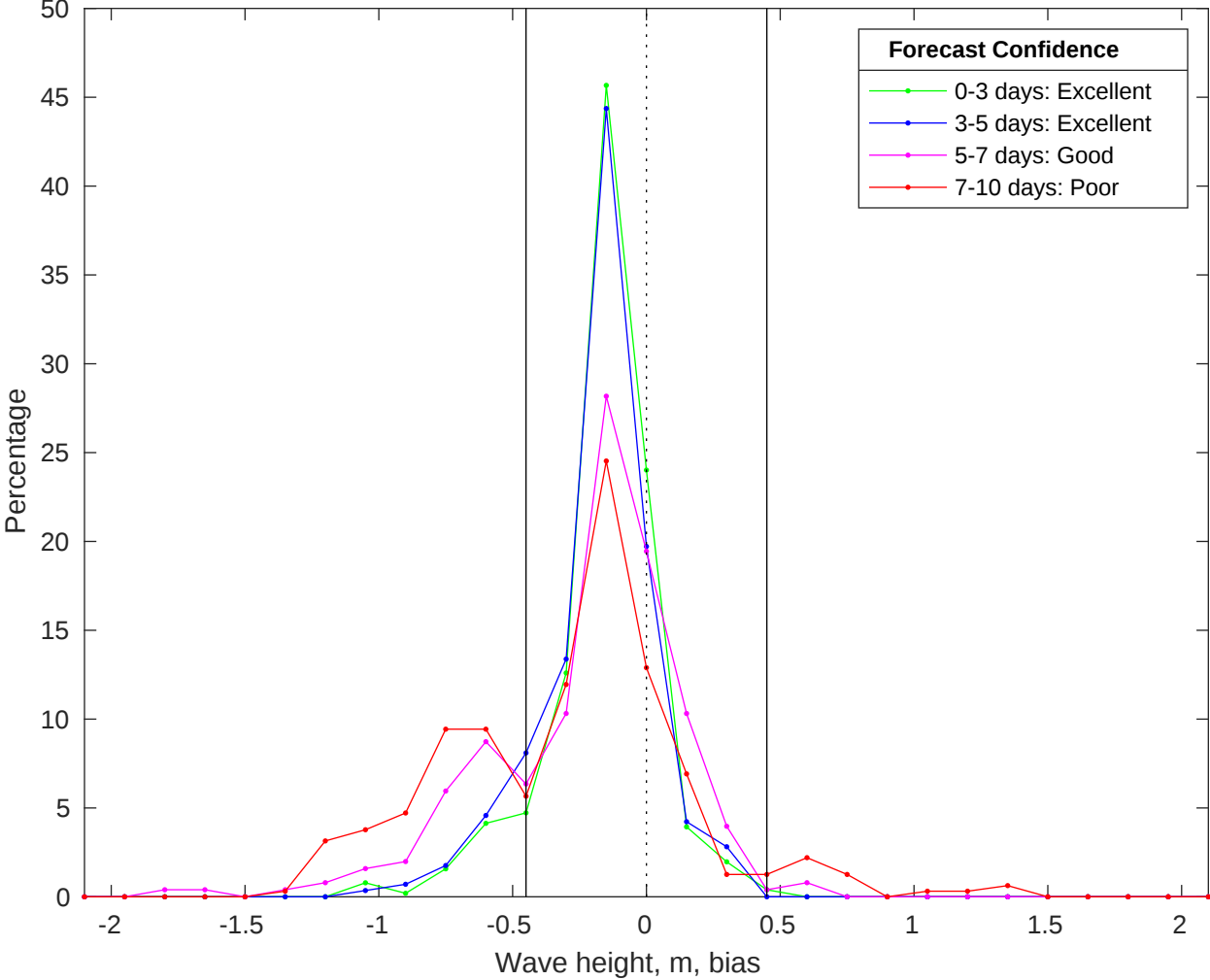
NDBC 42036 vs CMEMS Waves Bias Histogram: 05-Jan-2026
