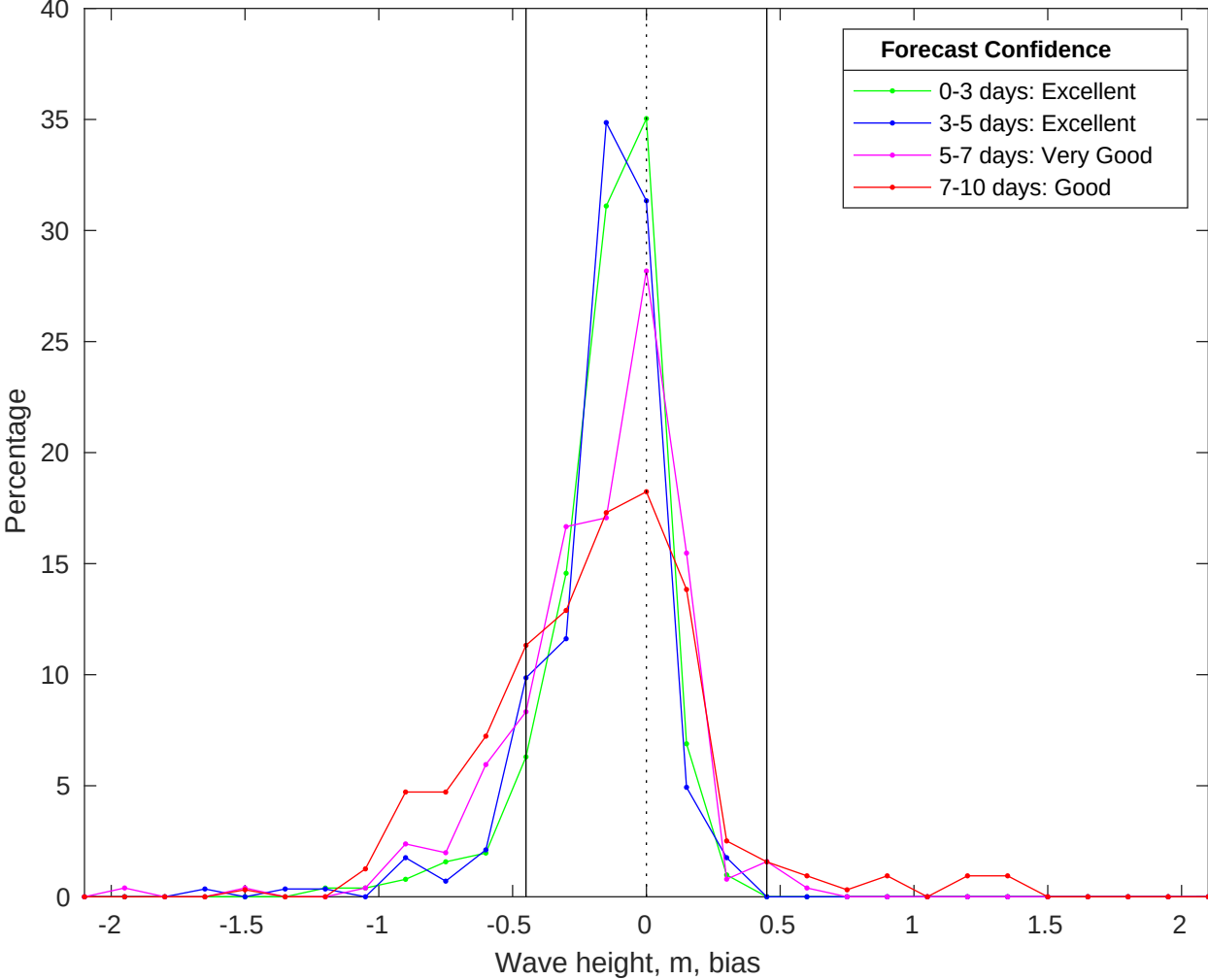
NDBC 42040 vs CMEMS Waves Bias Histogram: 05-Jan-2026
