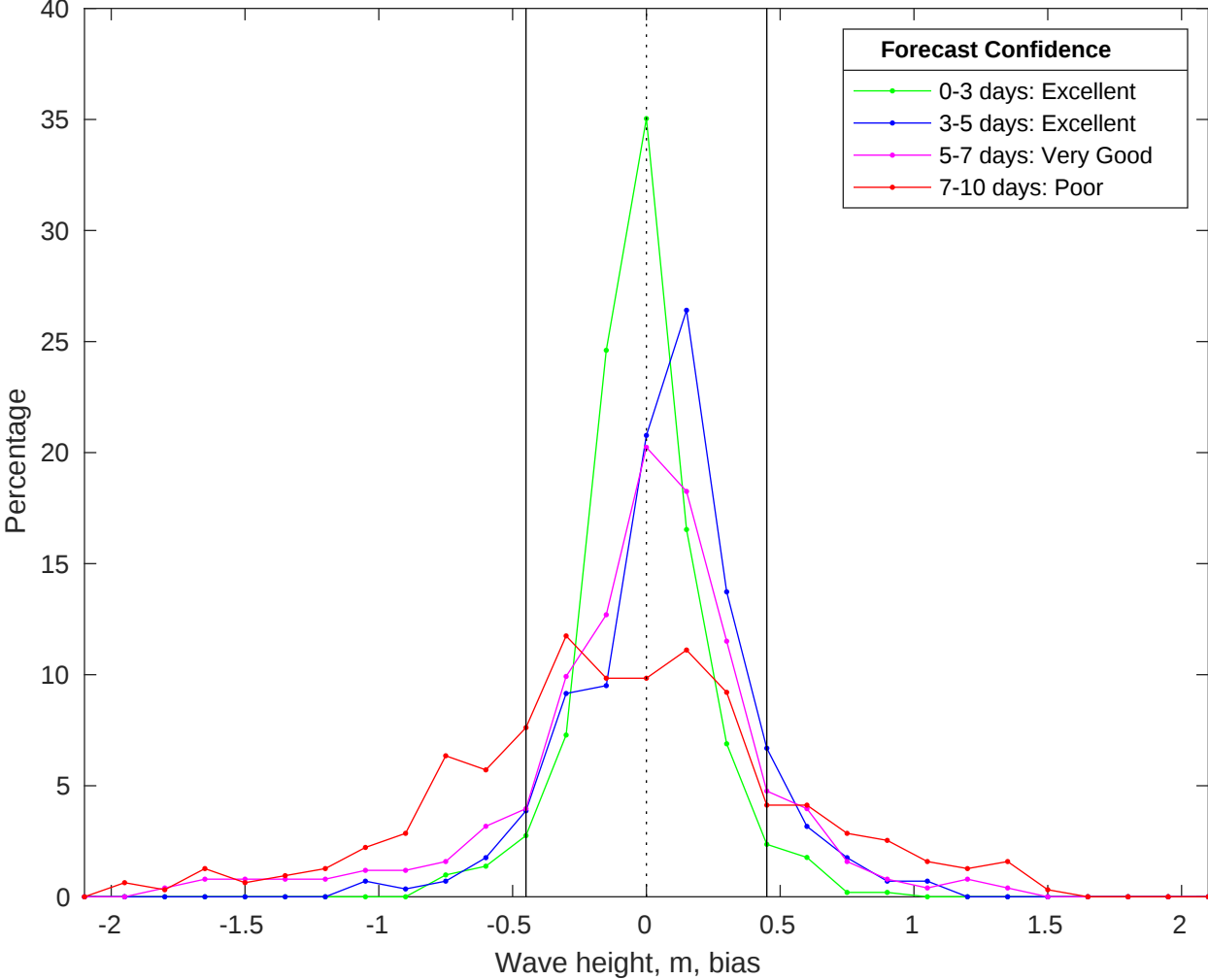
NDBC 46011 vs CMEMS Waves Bias Histogram: 05-Jan-2026
