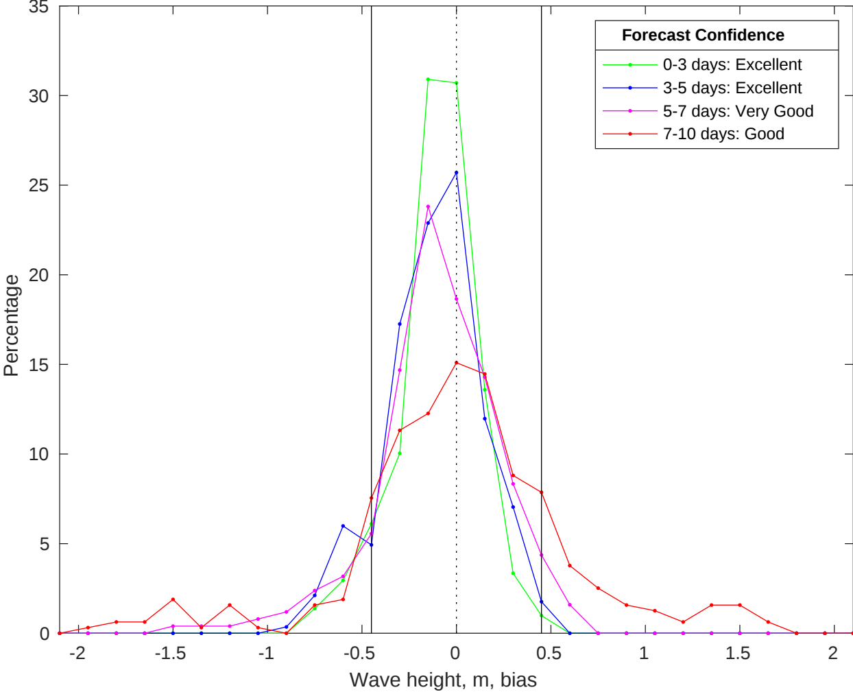
NDBC 51000 vs CMEMS Waves Bias Histogram: 05-Jan-2026
