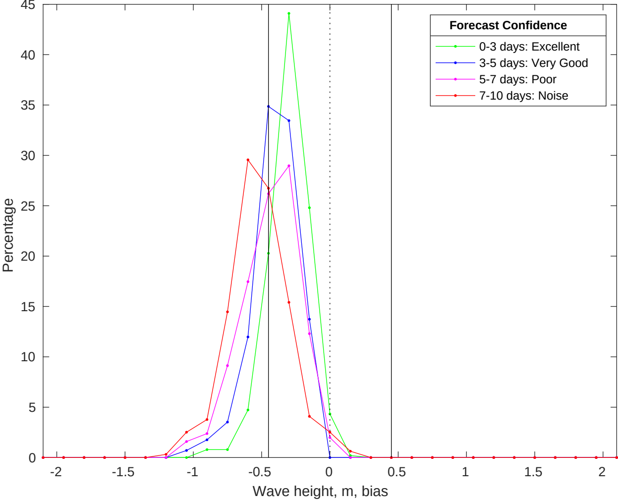
NDBC 51209 vs CMEMS Waves Bias Histogram: 05-Jan-2026
