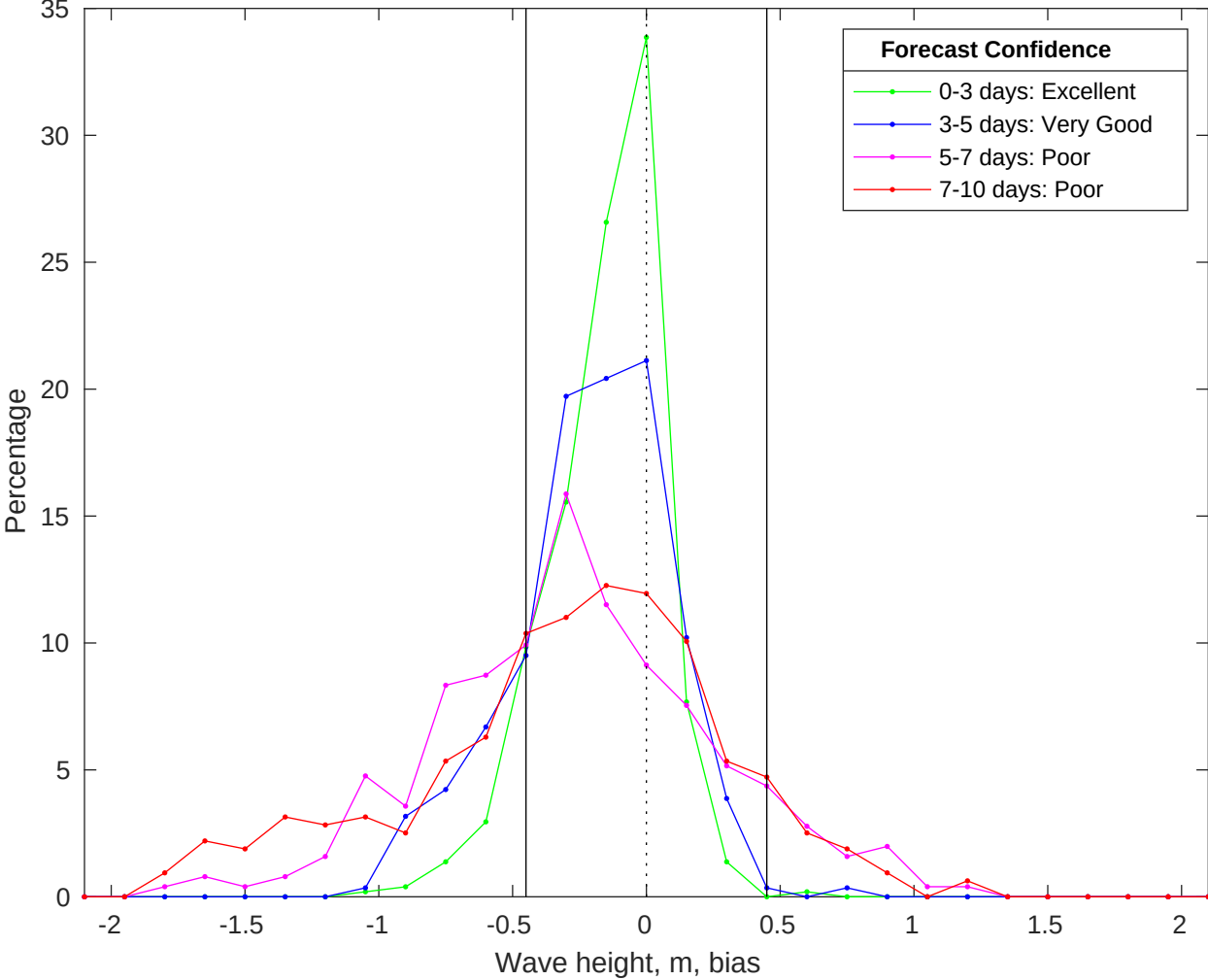
NDBC 41013 vs CMEMS Waves Bias Histogram: 07-Jan-2026
