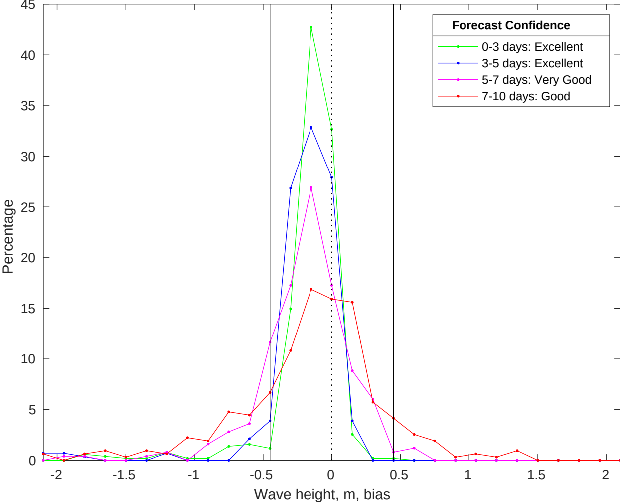
NDBC 42019 vs CMEMS Waves Bias Histogram: 07-Jan-2026
