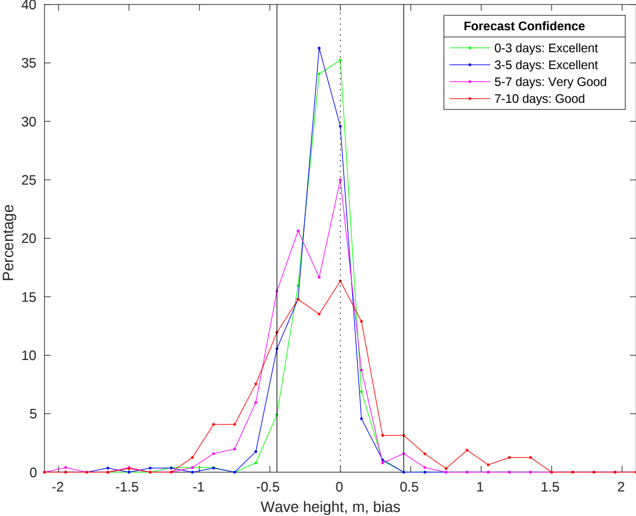
NDBC 42040 vs CMEMS Waves Bias Histogram: 07-Jan-2026
