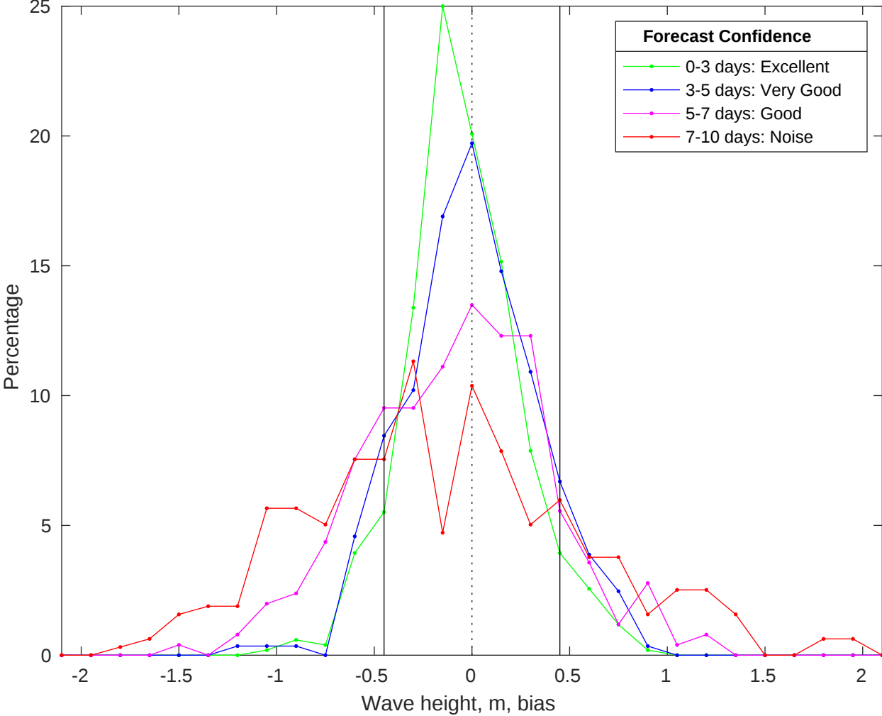
NDBC 46054 vs CMEMS Waves Bias Histogram: 07-Jan-2026
