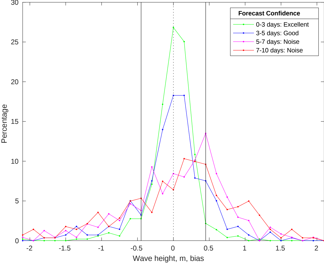
NDBC 46059 vs CMEMS Waves Bias Histogram: 07-Jan-2026
