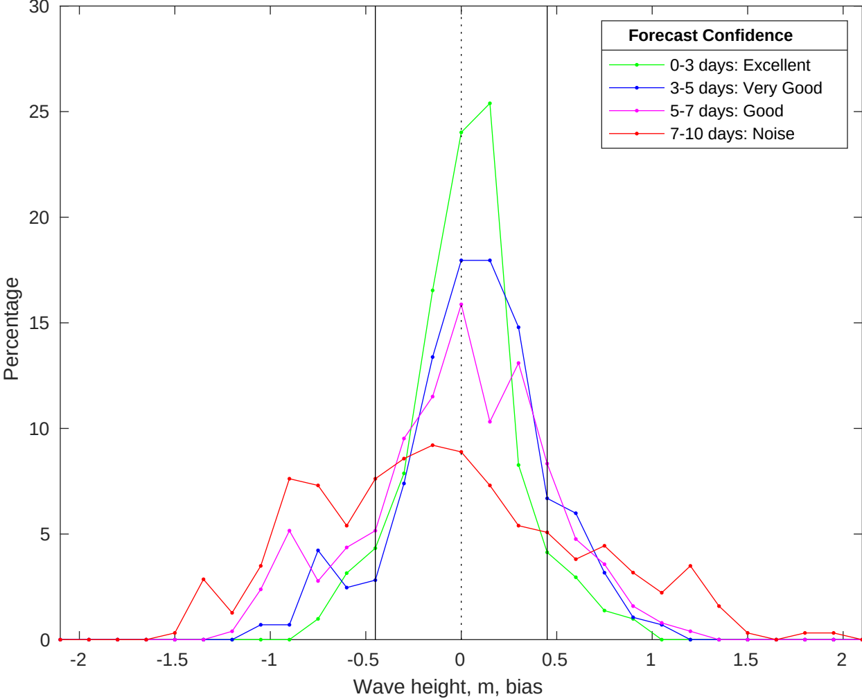
NDBC 46069 vs CMEMS Waves Bias Histogram: 07-Jan-2026
