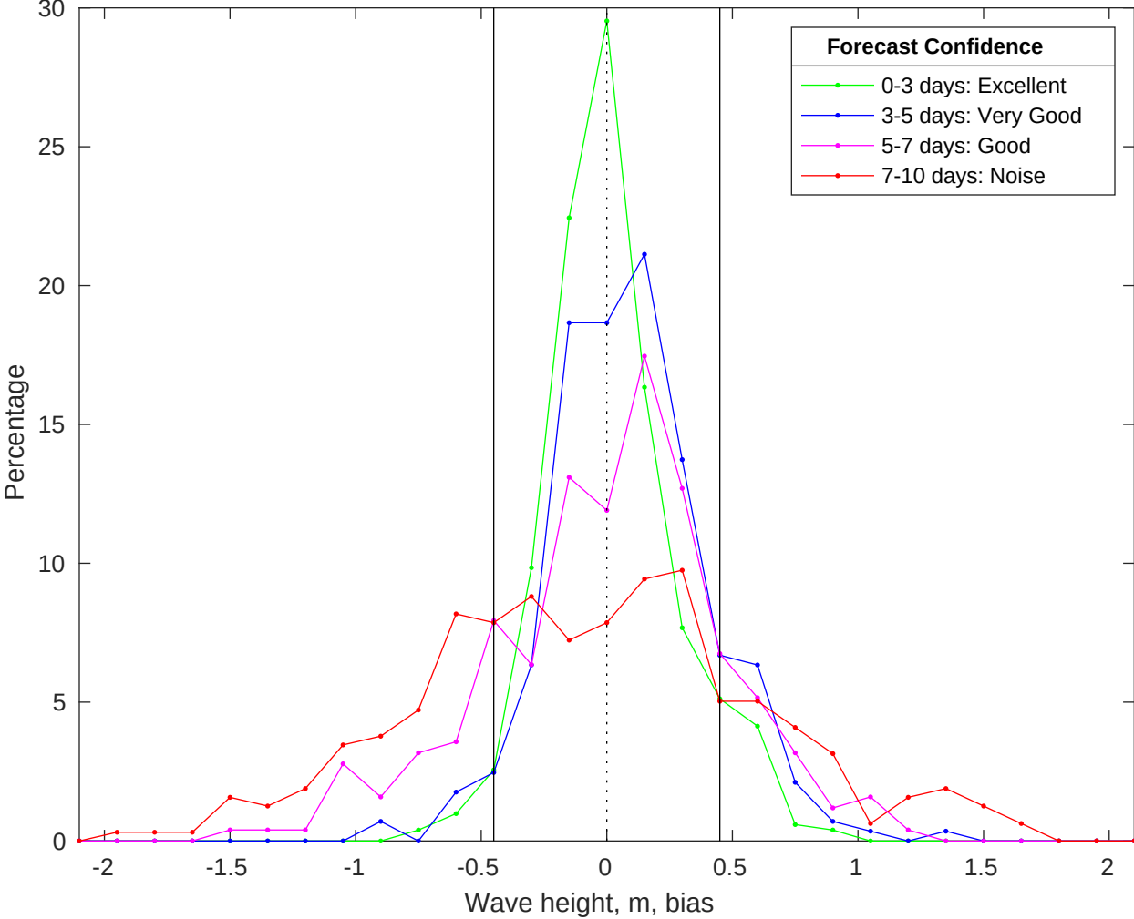
NDBC 46259 vs CMEMS Waves Bias Histogram: 07-Jan-2026
