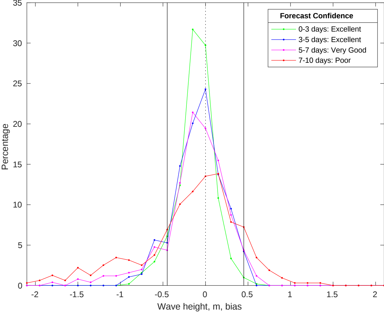
NDBC 51000 vs CMEMS Waves Bias Histogram: 07-Jan-2026
