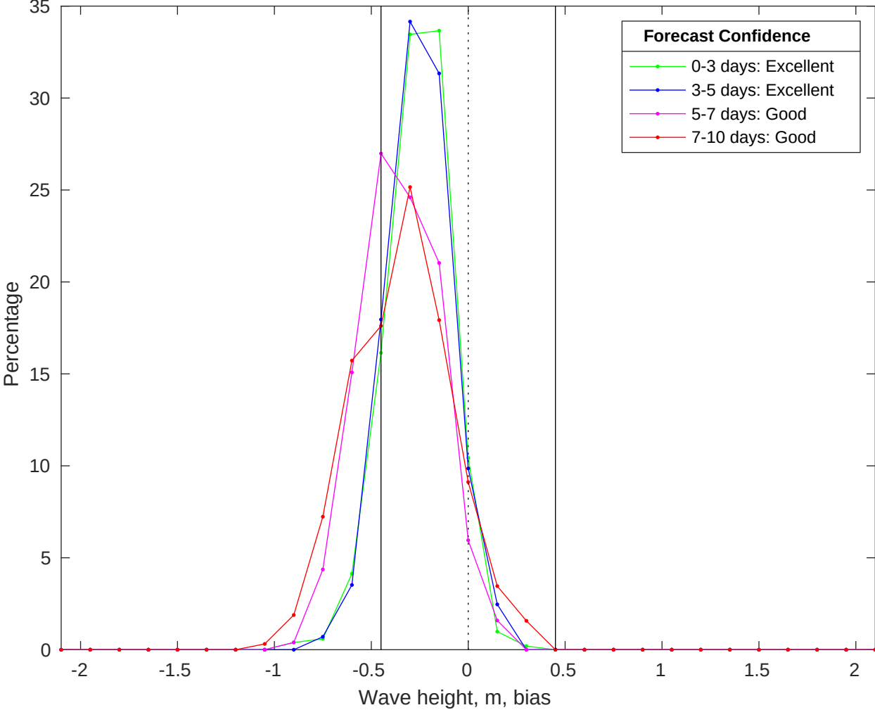
NDBC 52213 vs CMEMS Waves Bias Histogram: 07-Jan-2026
