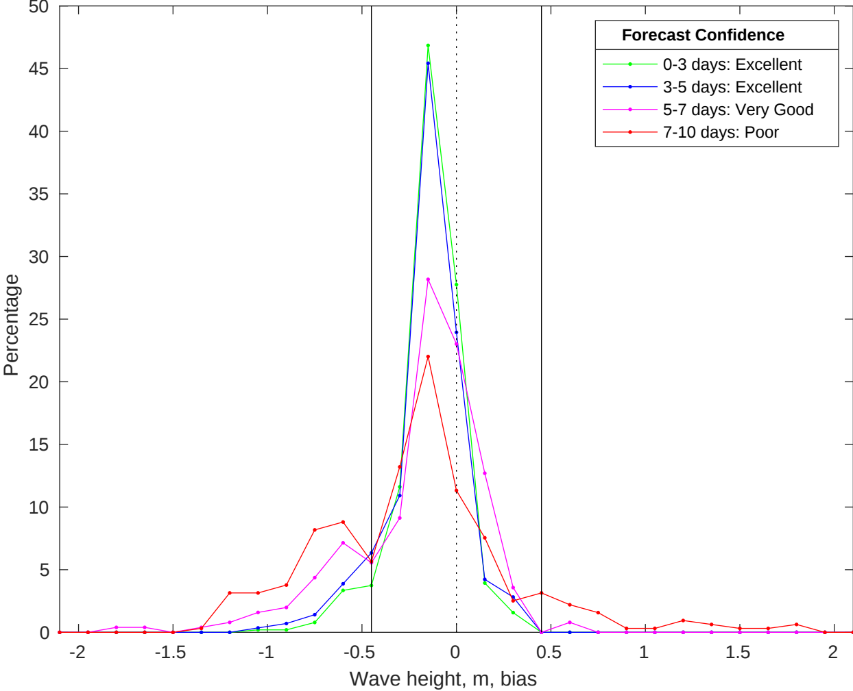
NDBC 42036 vs CMEMS Waves Bias Histogram: 08-Jan-2026
