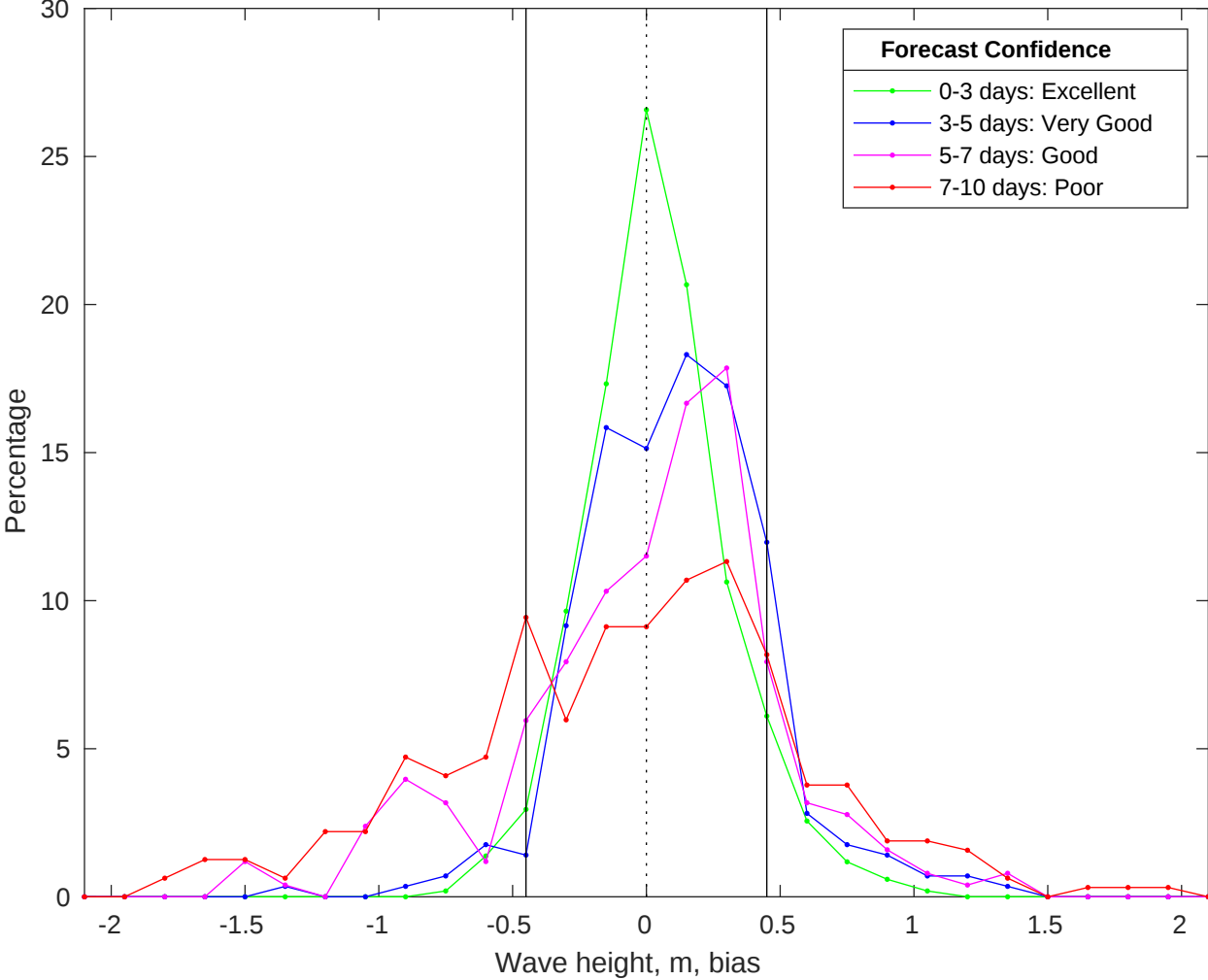
NDBC 46028 vs CMEMS Waves Bias Histogram: 08-Jan-2026
