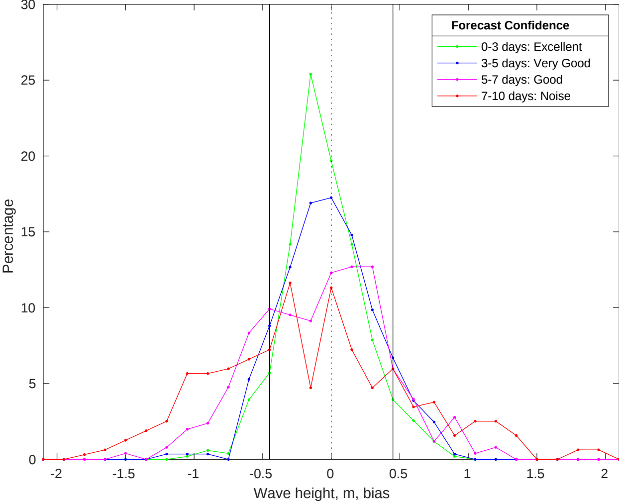
NDBC 46054 vs CMEMS Waves Bias Histogram: 08-Jan-2026
