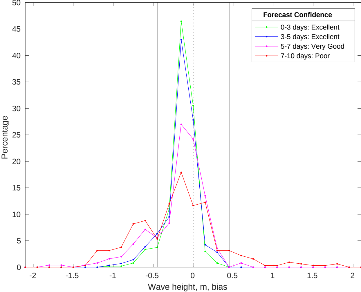
NDBC 42036 vs CMEMS Waves Bias Histogram: 09-Jan-2026
