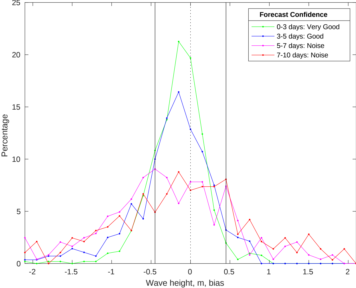
NDBC 44008 vs CMEMS Waves Bias Histogram: 09-Jan-2026
