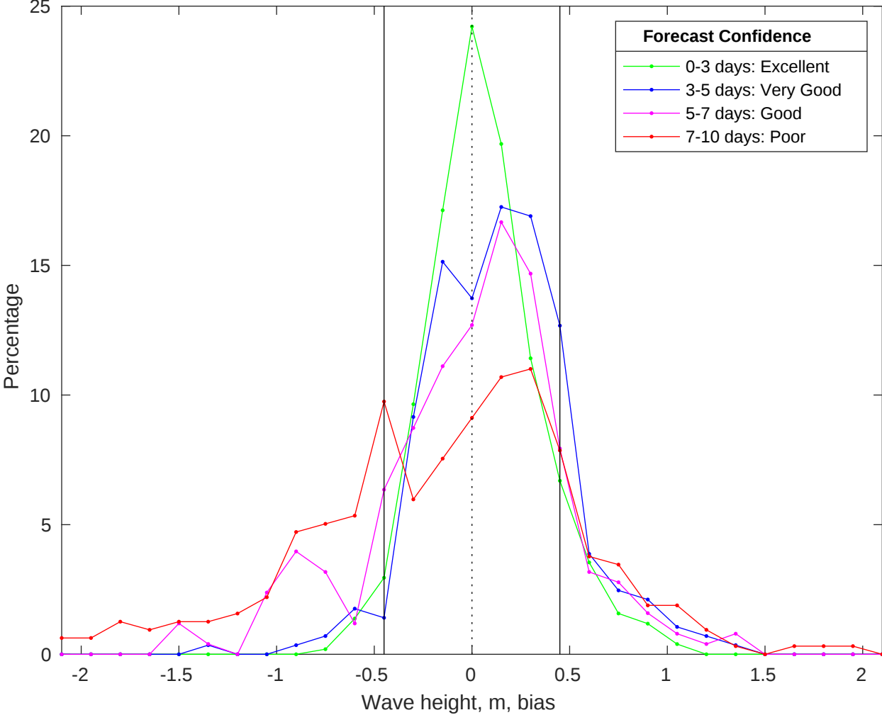
NDBC 46028 vs CMEMS Waves Bias Histogram: 09-Jan-2026
