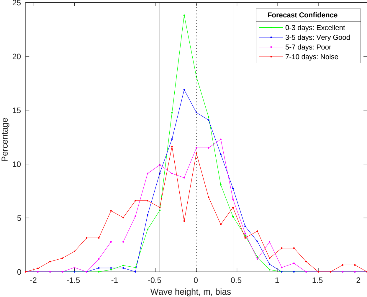
NDBC 46054 vs CMEMS Waves Bias Histogram: 09-Jan-2026
