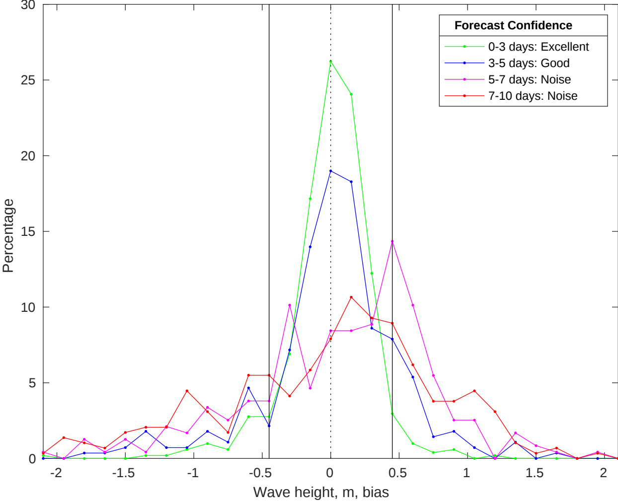
NDBC 46059 vs CMEMS Waves Bias Histogram: 09-Jan-2026
