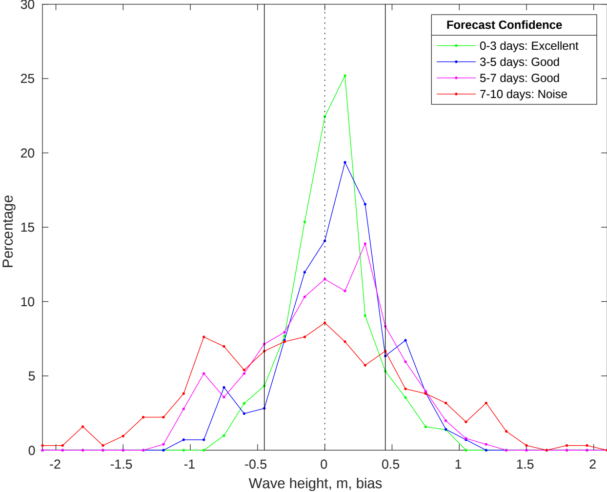
NDBC 46069 vs CMEMS Waves Bias Histogram: 09-Jan-2026
