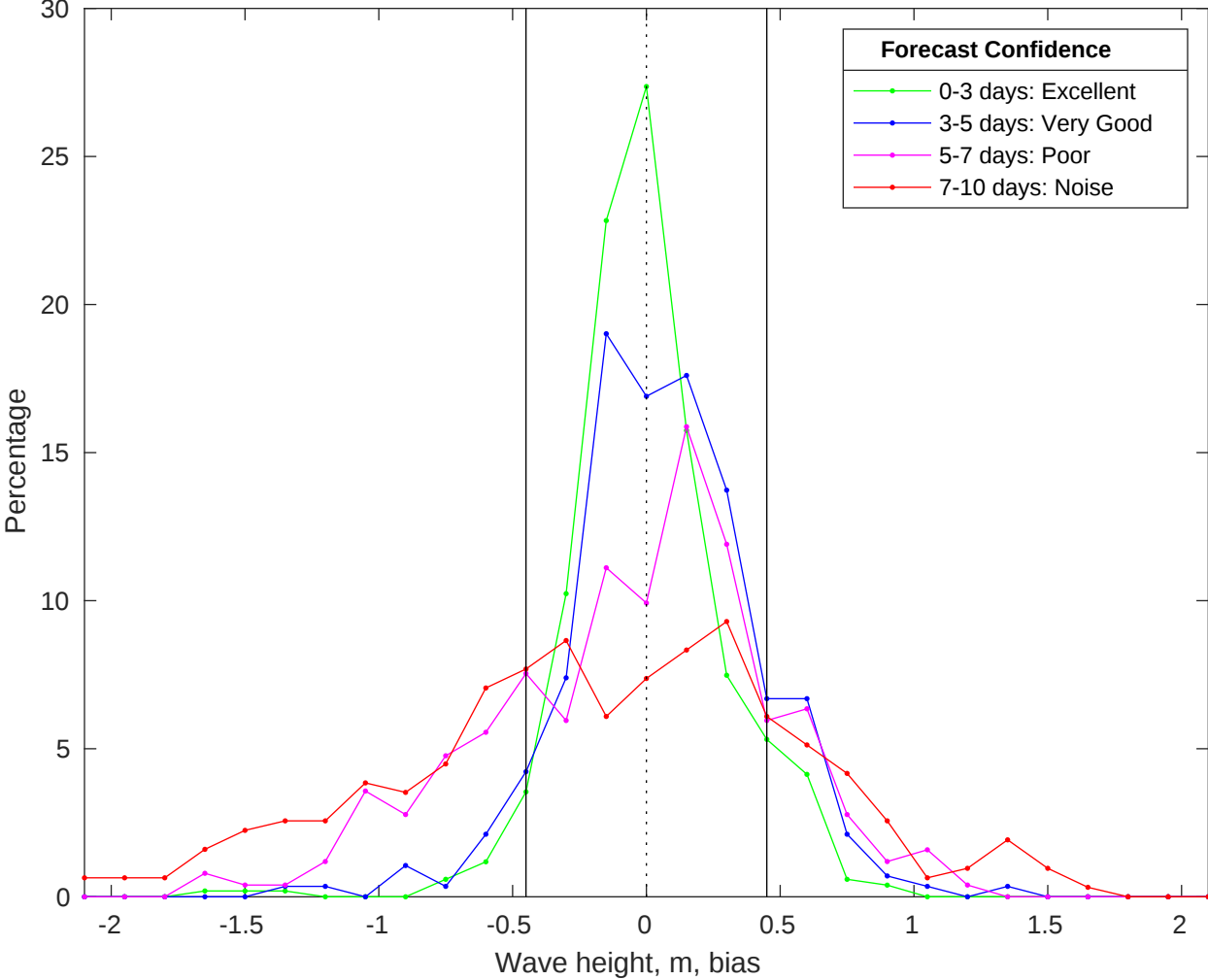
NDBC 46259 vs CMEMS Waves Bias Histogram: 09-Jan-2026
