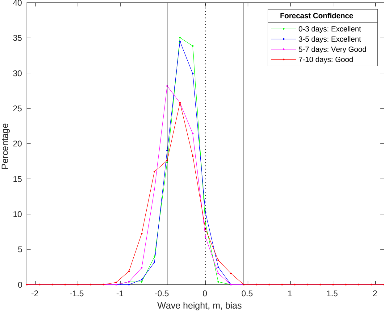
NDBC 52213 vs CMEMS Waves Bias Histogram: 09-Jan-2026
