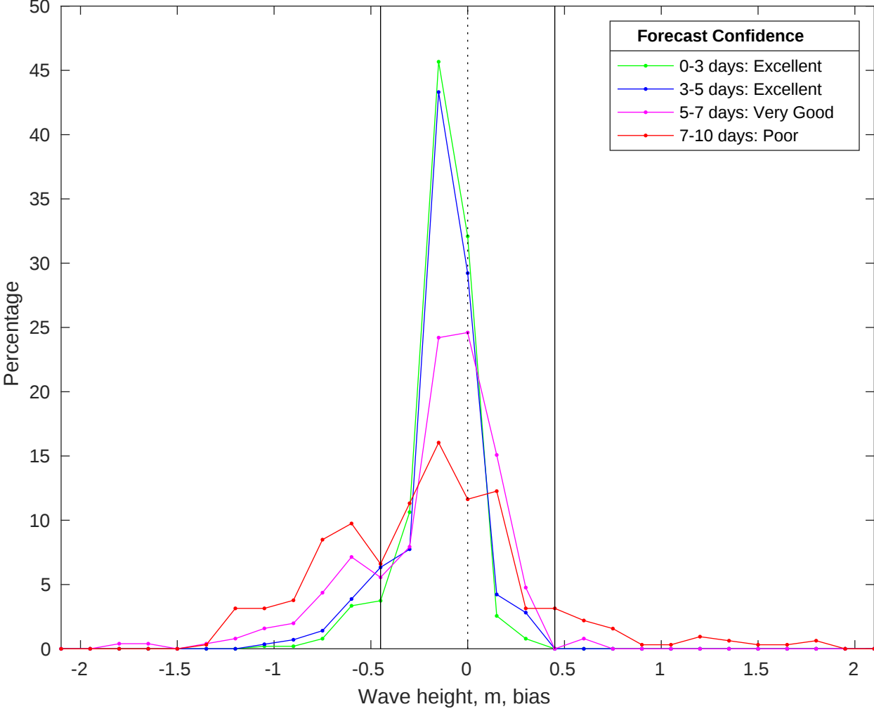
NDBC 42036 vs CMEMS Waves Bias Histogram: 10-Jan-2026
