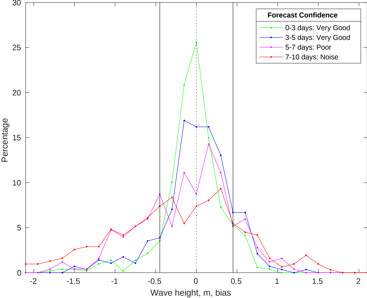
NDBC 46259 vs CMEMS Waves Bias Histogram: 10-Jan-2026
