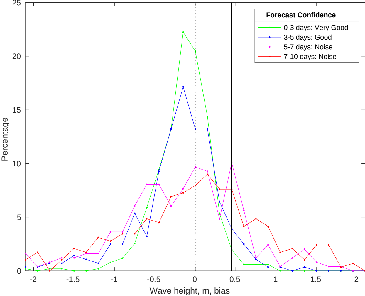
NDBC 44008 vs CMEMS Waves Bias Histogram: 11-Jan-2026
