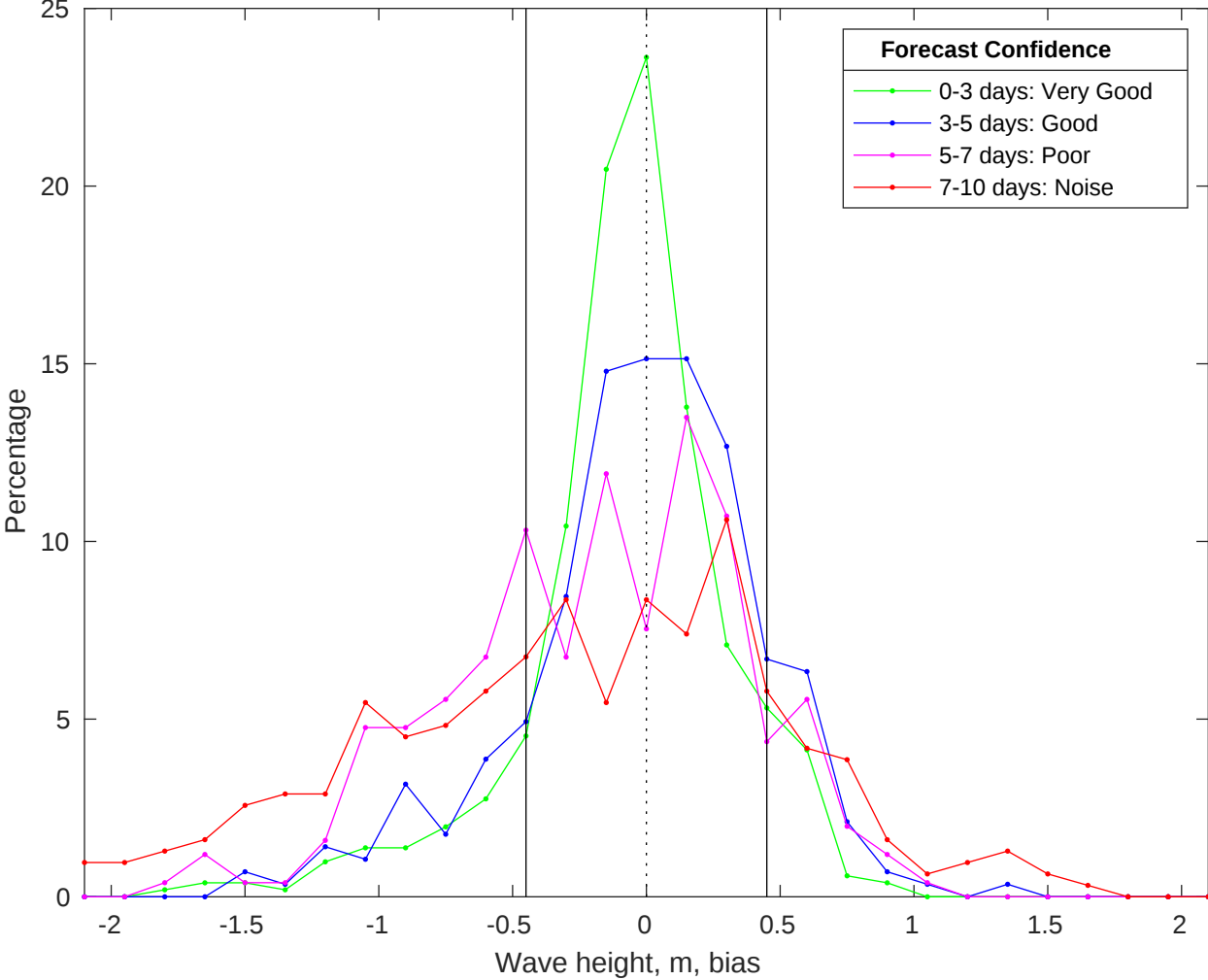
NDBC 46259 vs CMEMS Waves Bias Histogram: 11-Jan-2026
