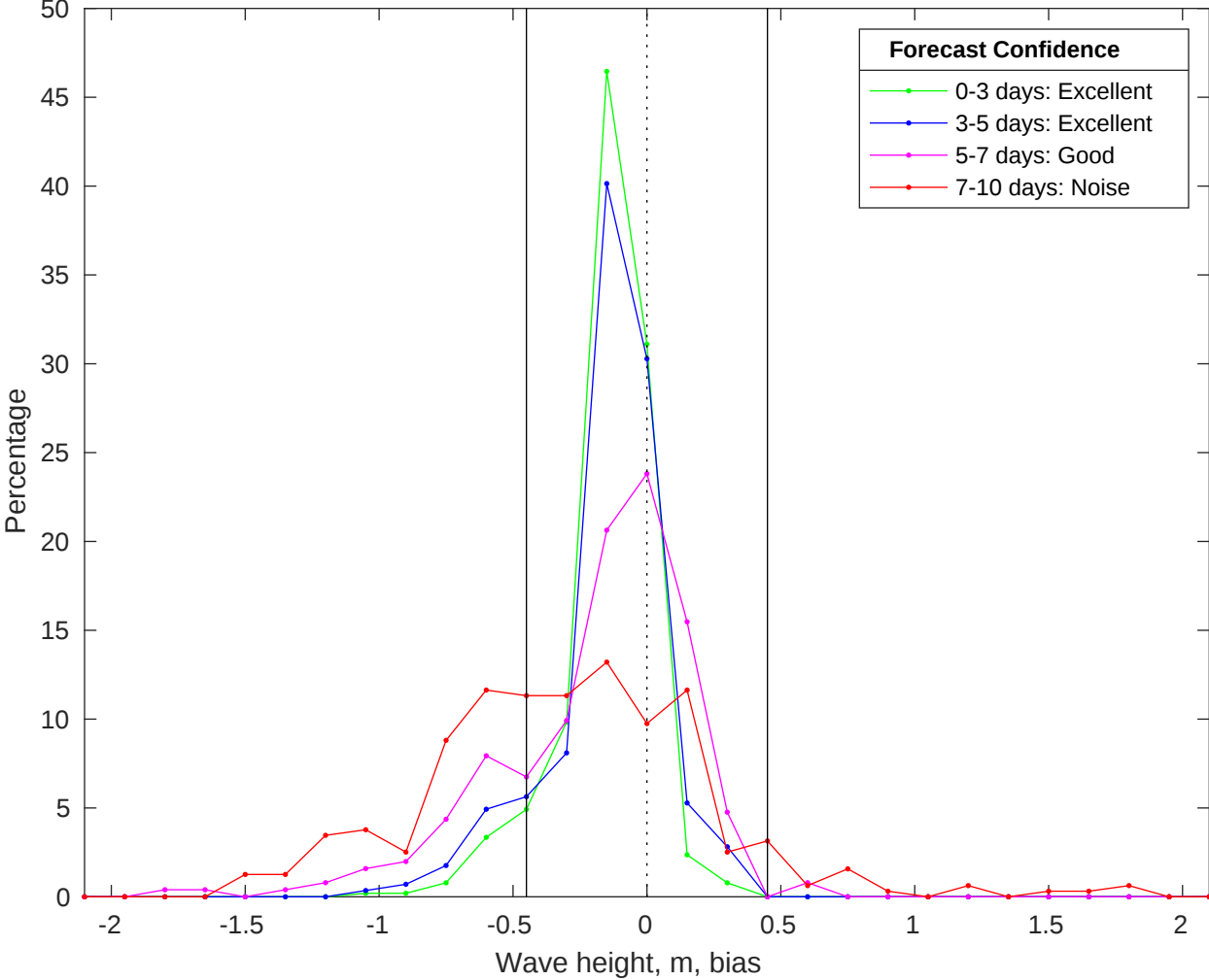
NDBC 42036 vs CMEMS Waves Bias Histogram: 12-Jan-2026
