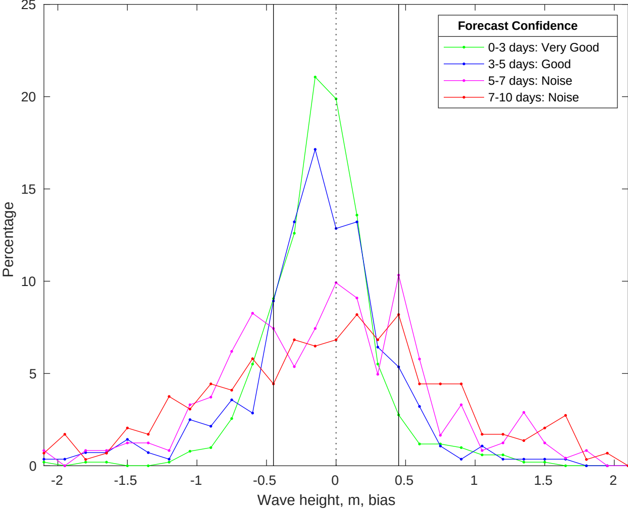
NDBC 44008 vs CMEMS Waves Bias Histogram: 12-Jan-2026
