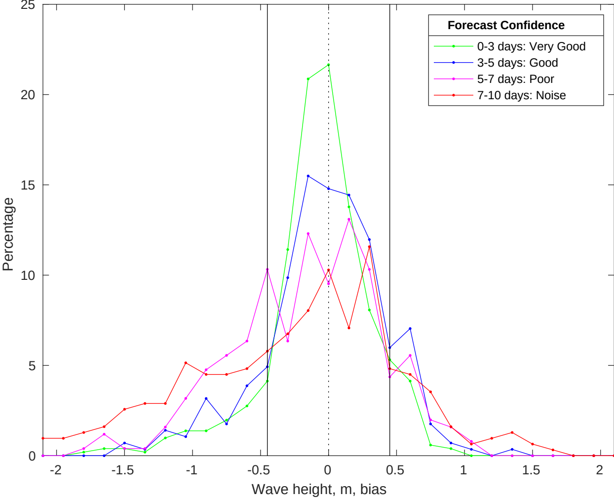
NDBC 46259 vs CMEMS Waves Bias Histogram: 12-Jan-2026
