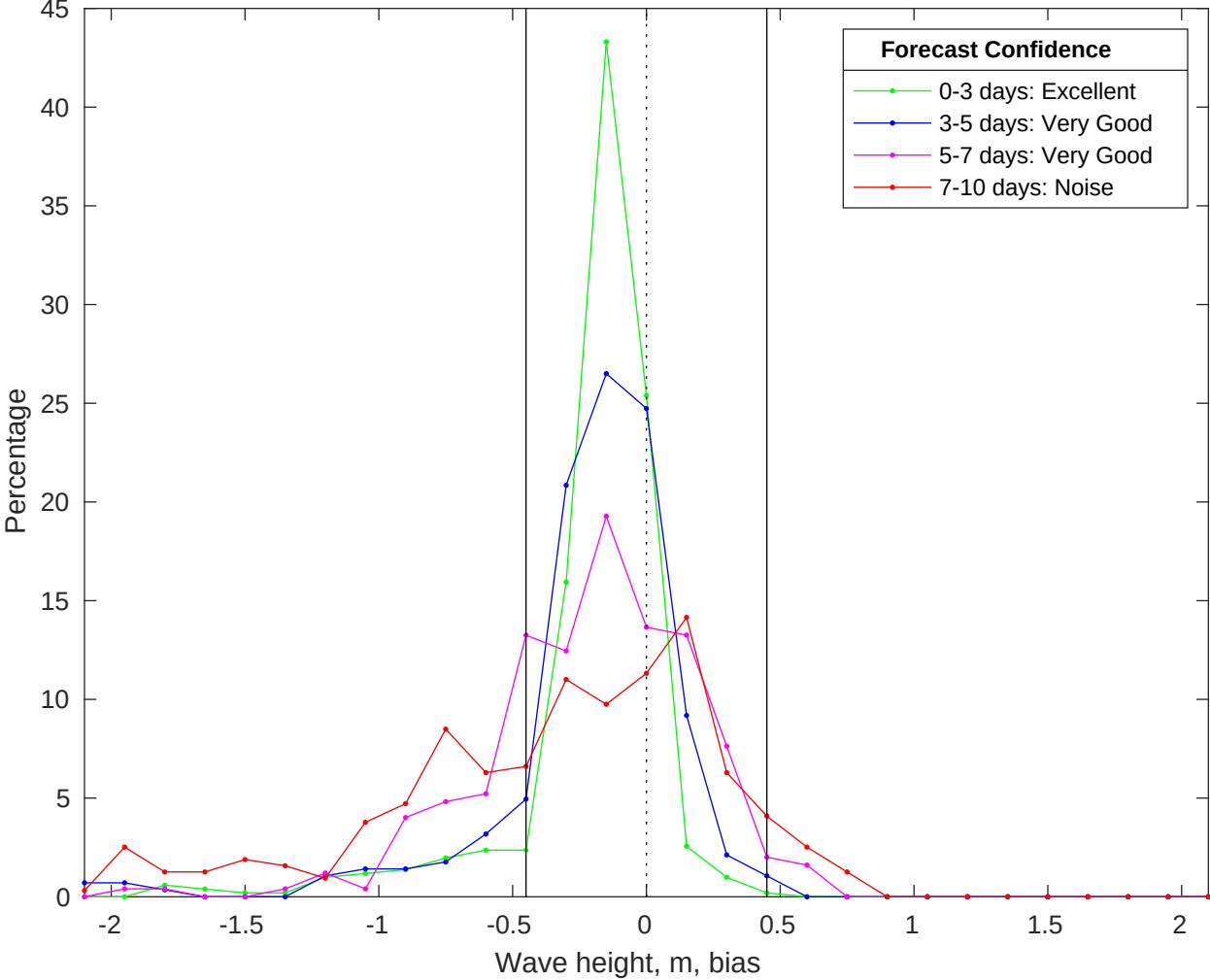
NDBC 42019 vs CMEMS Waves Bias Histogram: 13-Jan-2026
