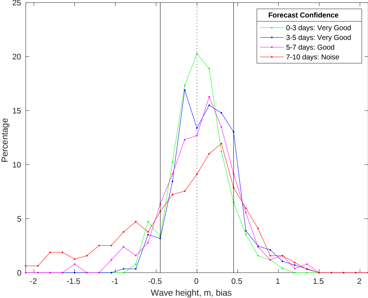
NDBC 46028 vs CMEMS Waves Bias Histogram: 13-Jan-2026
