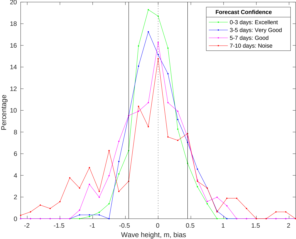
NDBC 46054 vs CMEMS Waves Bias Histogram: 13-Jan-2026
