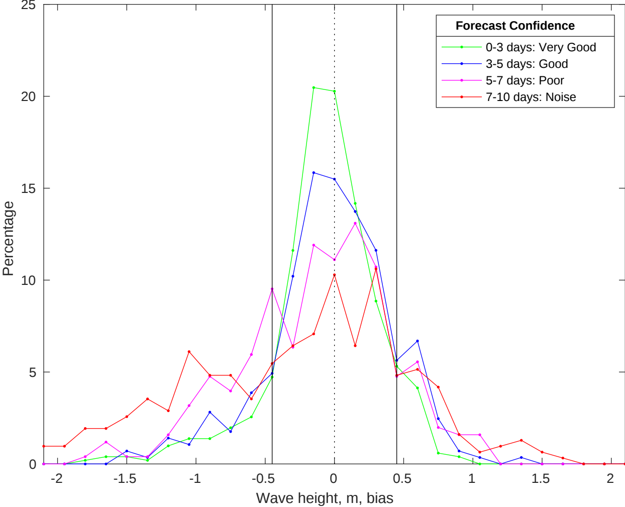
NDBC 46259 vs CMEMS Waves Bias Histogram: 13-Jan-2026
